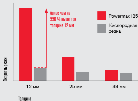
Относительная производительность резки низкоуглеродистой стали
